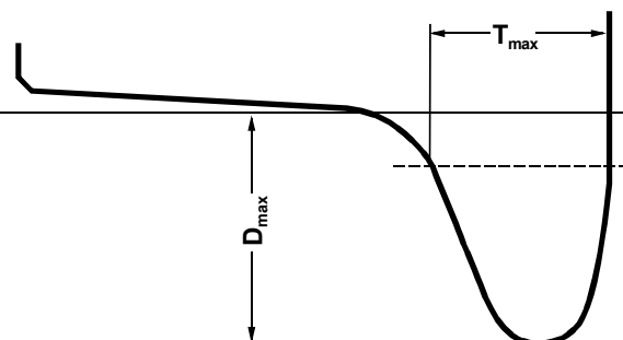
Abb. 3: Maximaler Spurkranz
